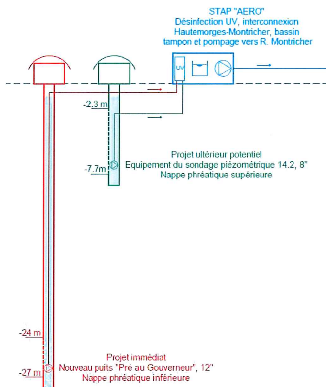
Schéma du futur puits « Pré au Gouverneur » (en rouge)
