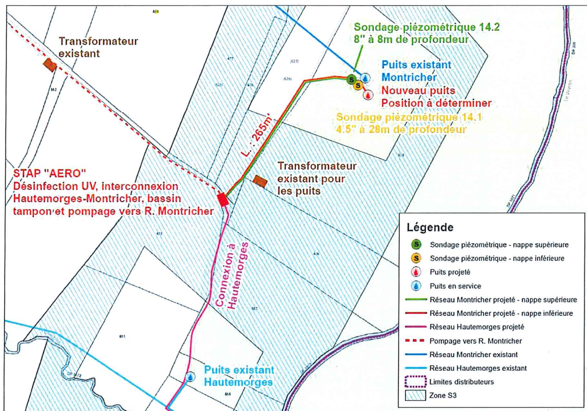
Situation du futur puits du « Pré au Gouverneur », de la future STAP AERO et des conduites de liaison
